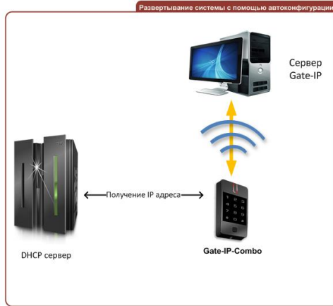
Рис.7. Автоконфигурация устройства
