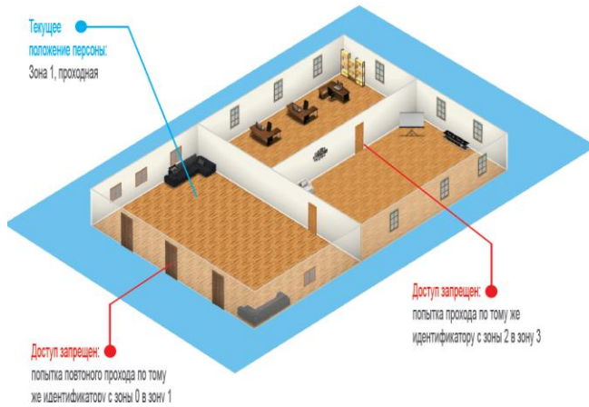
Рис 9. Отслеживание нарушений
