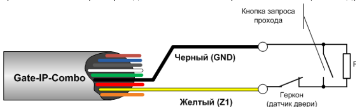
Рис.17. Подключение комбинированного шлейфа
